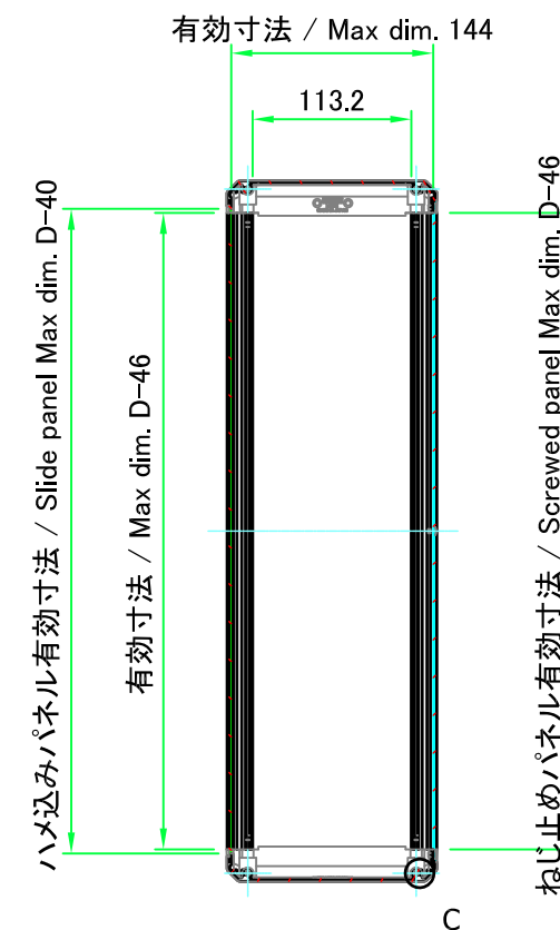
B-B ( 1 : 6 )
