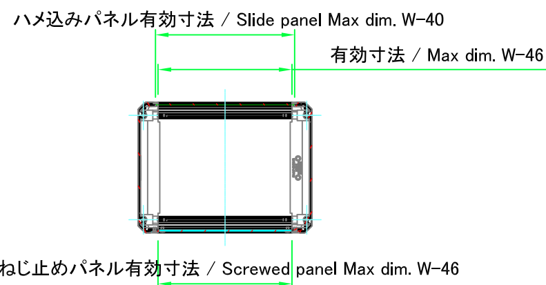
A-A ( 1 : 6 )
